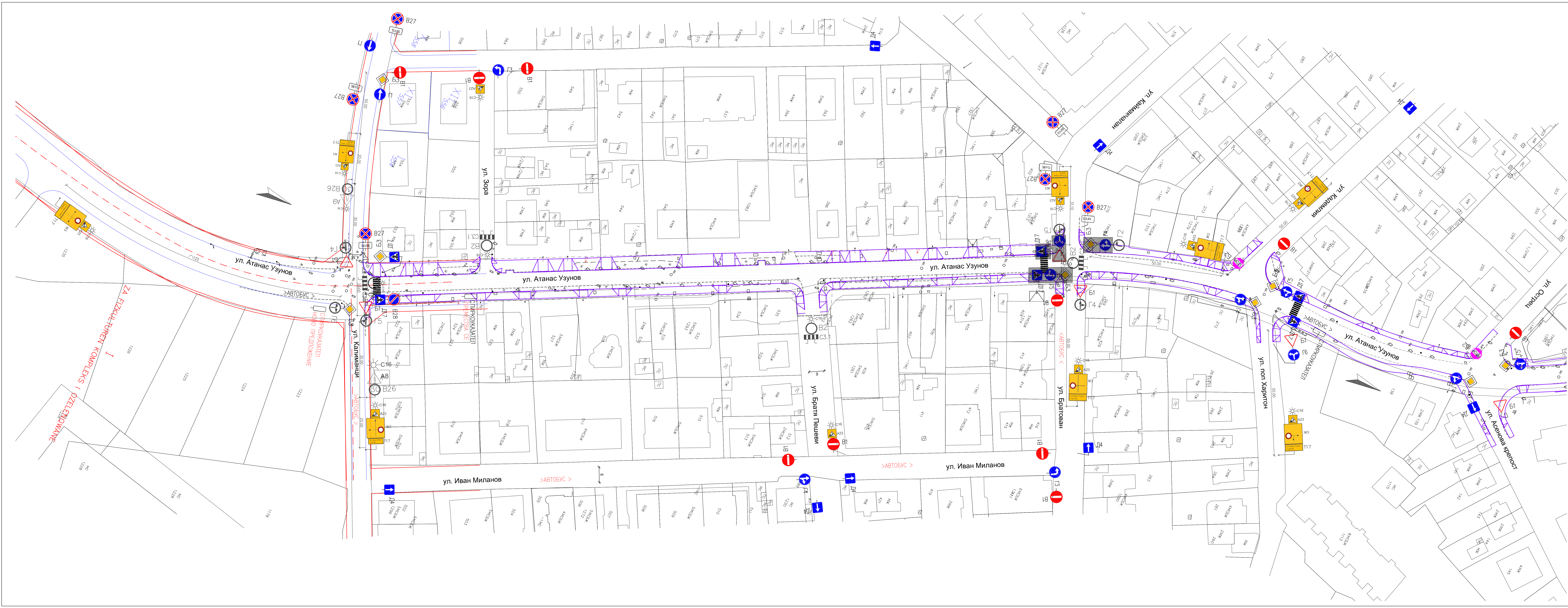
Работен участък 1—ул.Атанас Узунов, между ул.Калиманци и ул.Братован М 1:500
